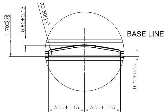
DETAIL B SCALE : 8 : 1
