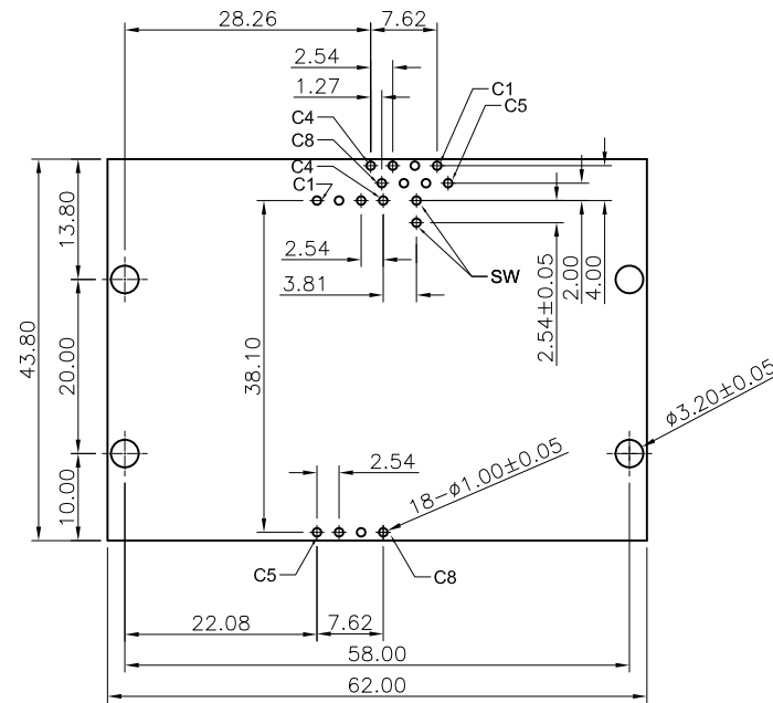
RECOMMEND P.C.B LAYOUT
