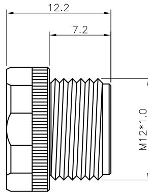
NUT
