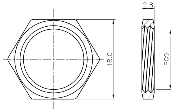
NUT
